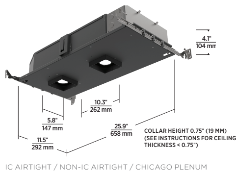
IC AIRTIGHT / NON-IC AIRTIGHT / CHICAGO PLENUM
