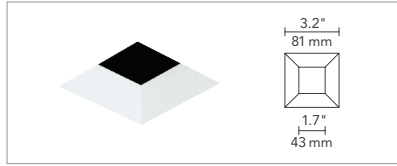
FLANGELESS BEVEL
